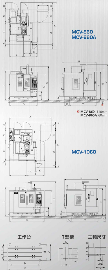
外型尺寸
