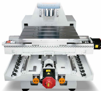
Y軸大跨距
